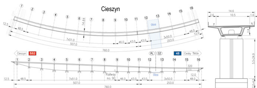
Ryc. 7. Most graniczny w Cieszynie
