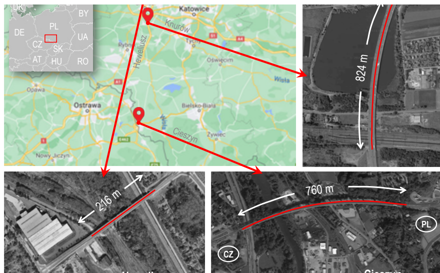
Ryc. 6. Mosty polygonowe do testowania aplikacji podczas inspekcji
