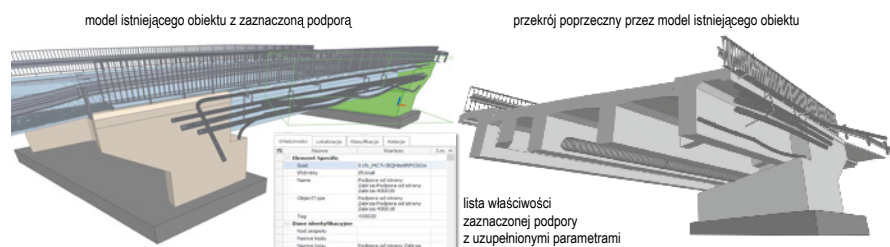
Ryc. 10. Model BIM mostu na Kłodnicy w Gliwicach
